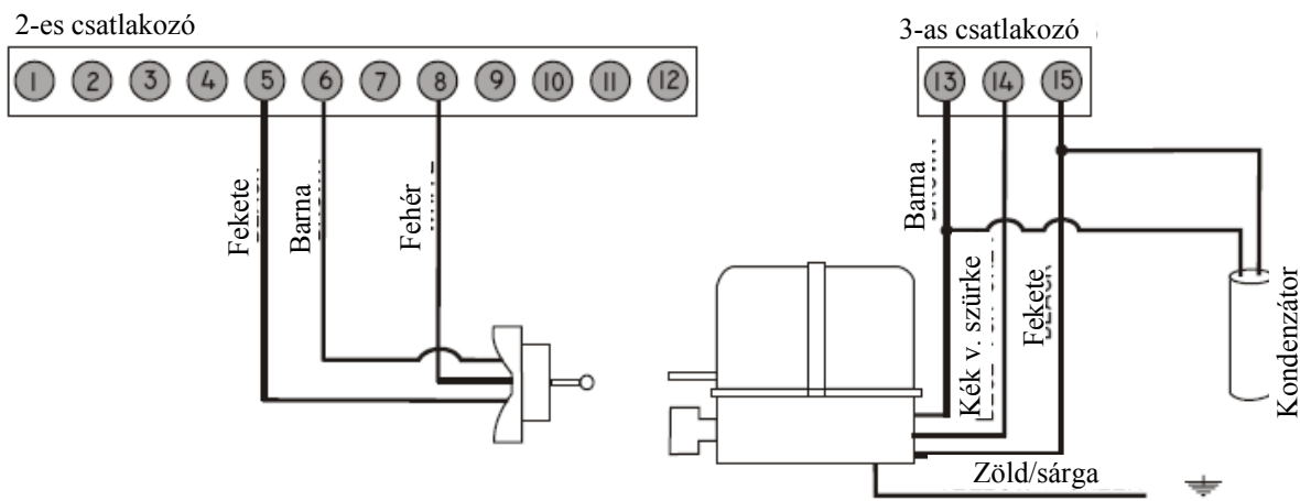
Baloldali szerelés (belső oldalról nézve)
